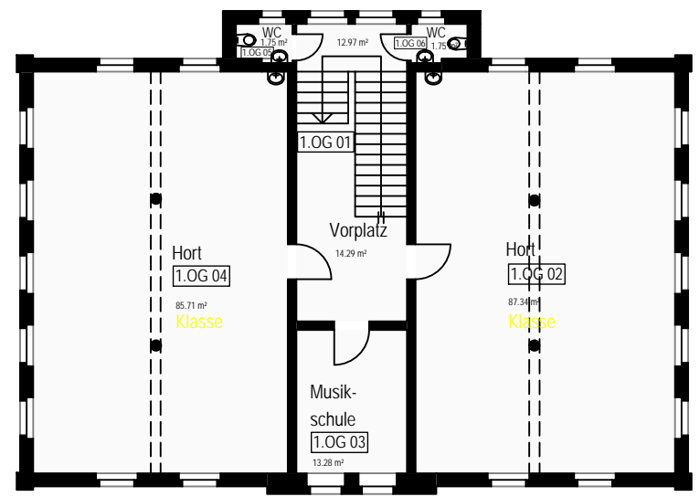
Grundriss 1. Obergeschoss
