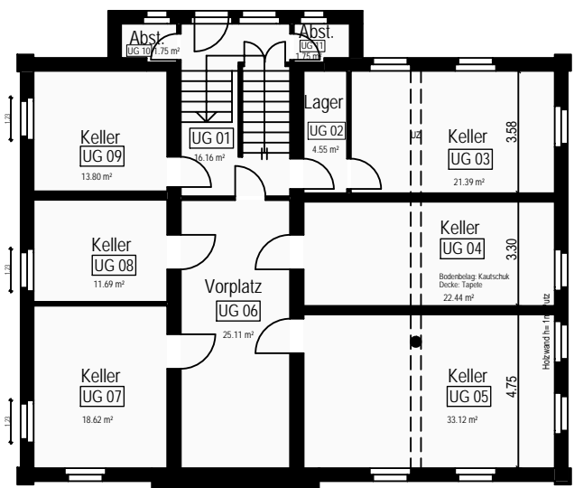
Grundriss Untergeschoss
